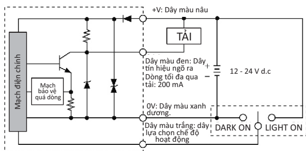
Mạch điện phía trong ← Cách kết nối phía bên ngoài
