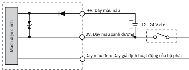
Mạch điện phía trong ← Cách kết nối phía bên ngoài
